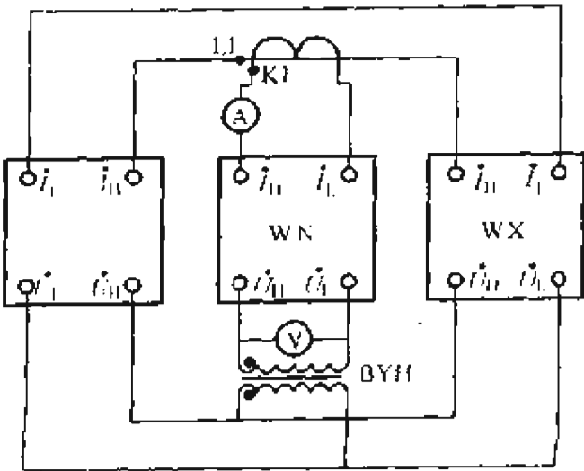
图 A.1 单相电能表检定接线图
