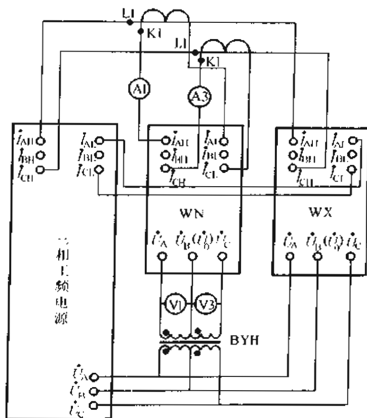
图 A.2 三相三线电能表检定接线图
