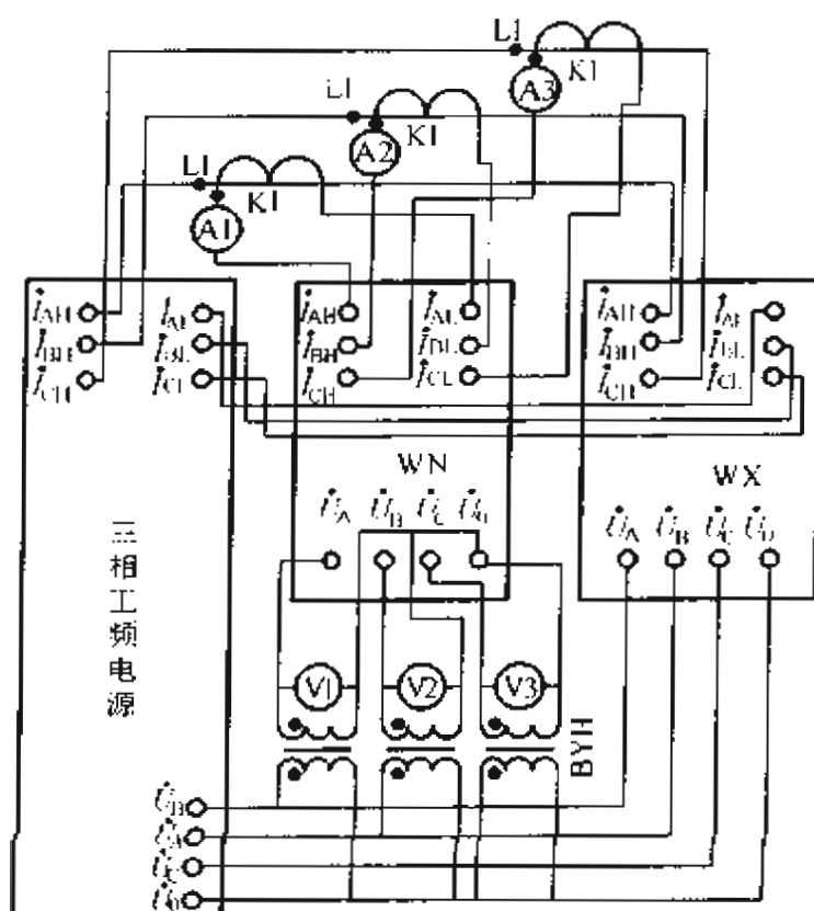
图 A.3 三相四线电能表检定接线图
